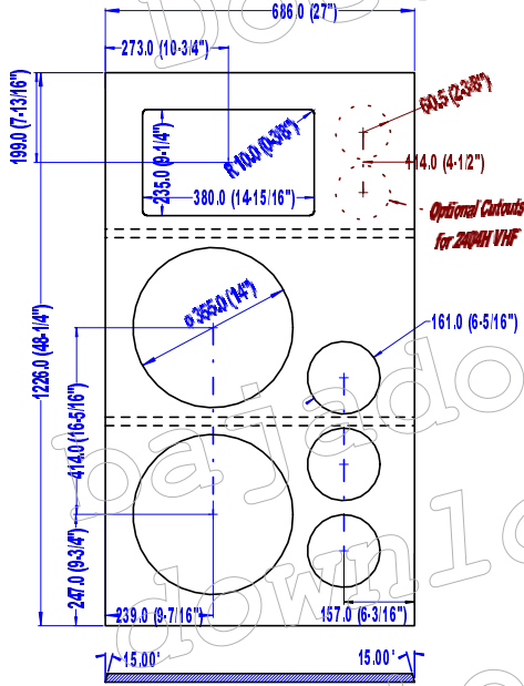
Baffle
